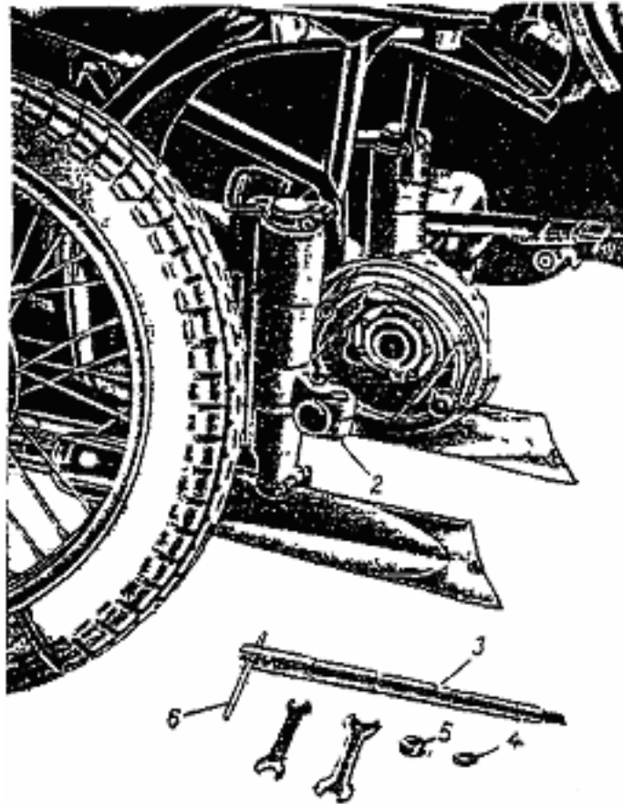
Bild 21 Abnehmen des Hinterrades
