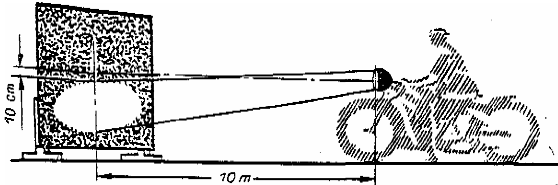
Bild 31 Skizze zur Einstellung des Scheinwerfers
