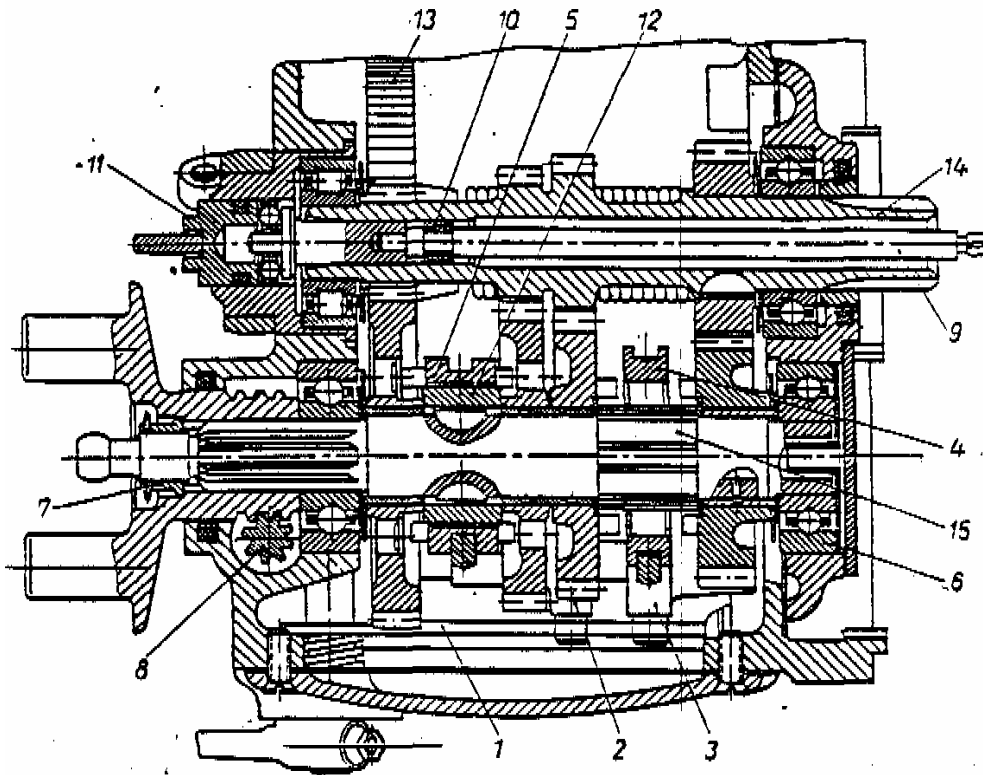
Bild 12 Das Getriebe
