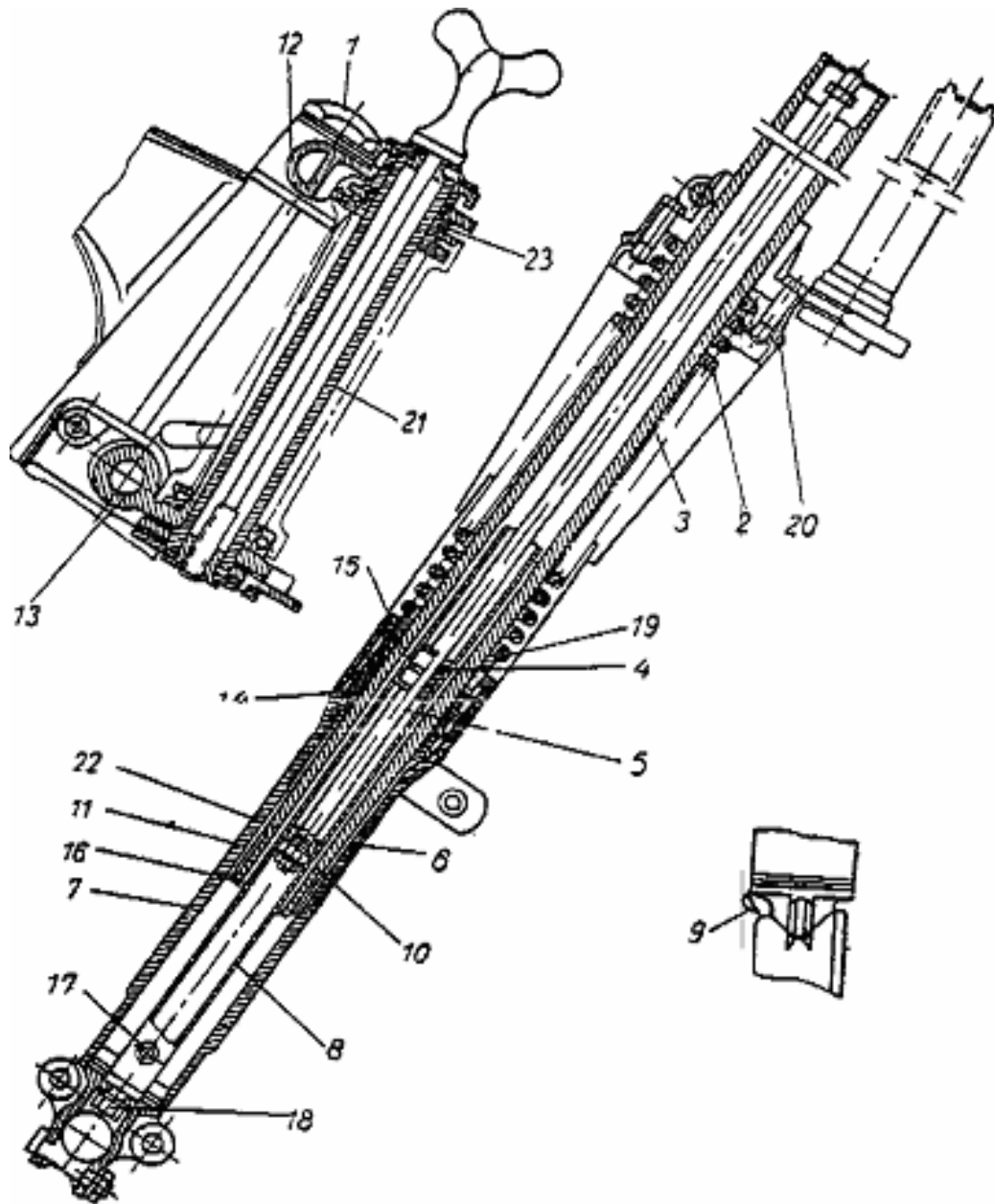
Bild 16 Die Vorderradgabel (Längsschnitt)
