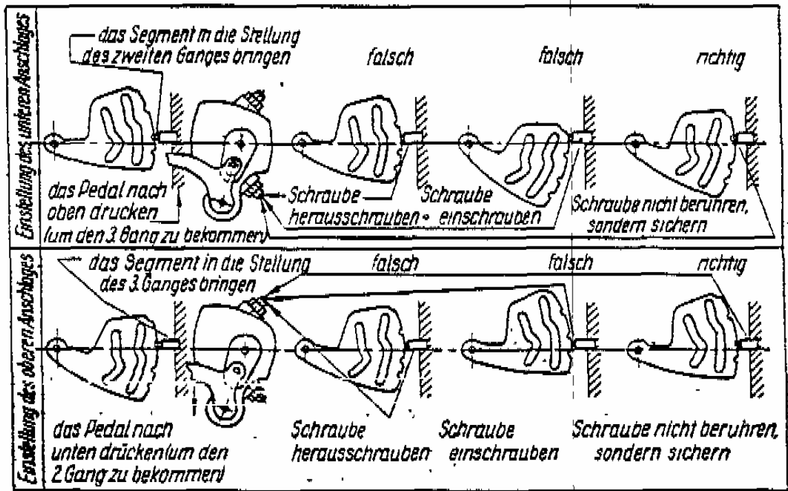
Bild 13 Einstellung des Getriebes
