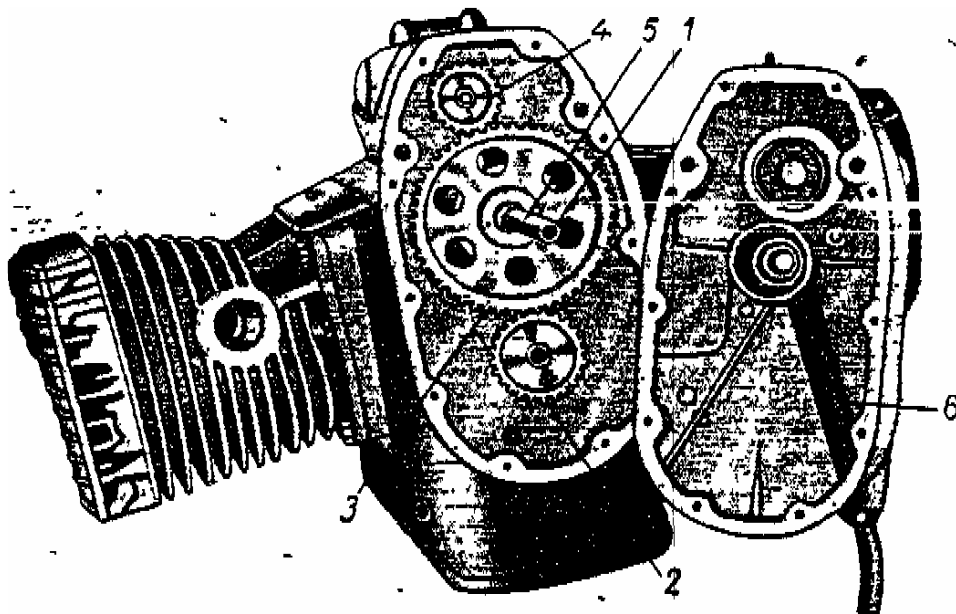
Bild 10 Einstellung der Nockenwelle
