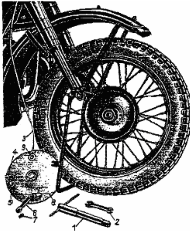
Bild 20 Abnehmen des Vorderrades
