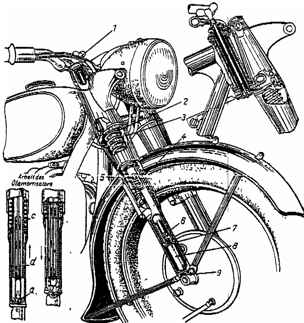
Bild 15 Die Vordergabel
