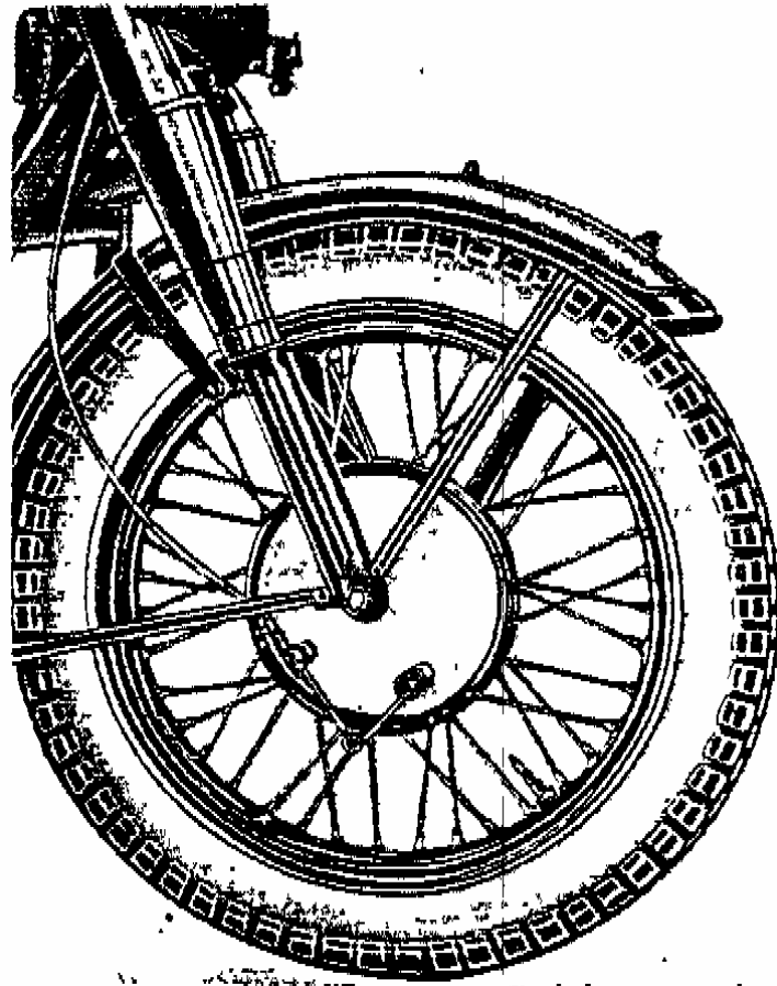
Bild 19 Einstellung der Vorderradbremse
