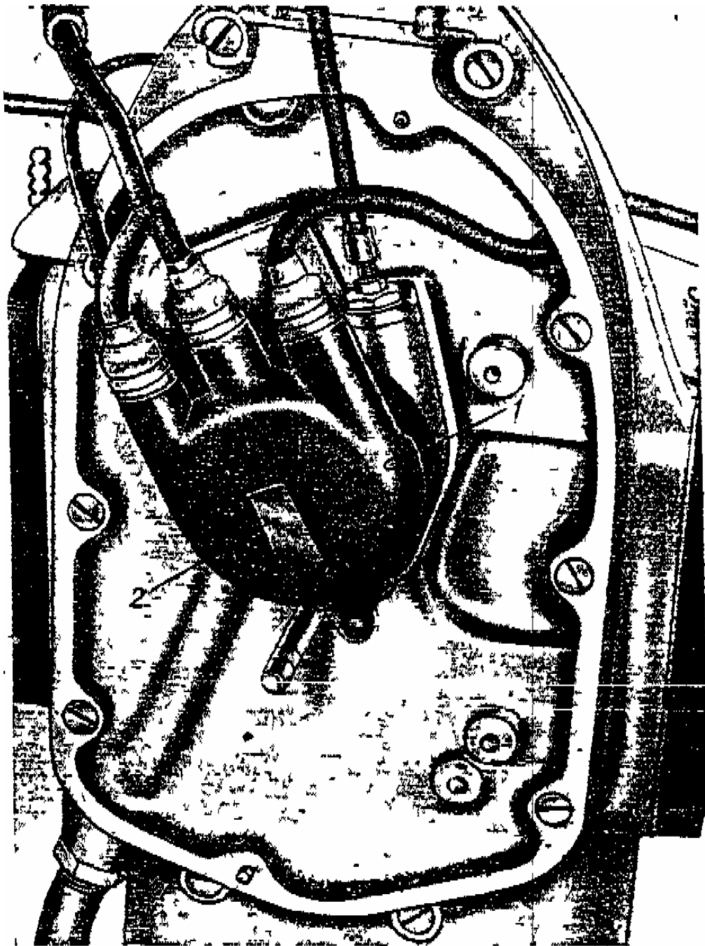
Bild 28 Die Lage des Verteilers PM — 05
